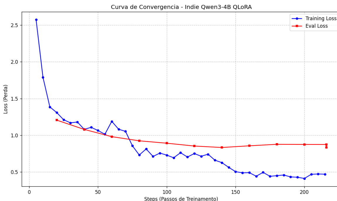
Figura 1. Perda de treino (azul) e de validação (vermelho) por passo. O ponto isolado no passo 216 é a avaliação do melhor checkpoint já restaurado.
